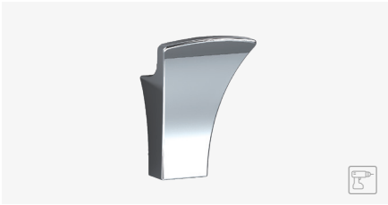
ROBEHOOK S7 ● CHROME A: 46 mm. B: 74 mm. C: 44 mm.
